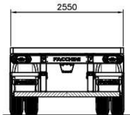
VISTA TRASEIRA
